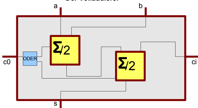
Der Volladdierer
