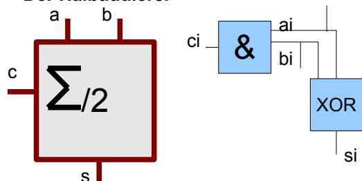
Der Halbaddierer
